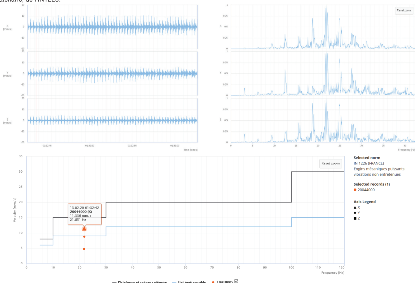
Figure 7. Signal temporel d'un événement, 3 axes orthogonaux, avec la transformée de Fourier. Le spectre fréquentiel dominant est bien autour de la plage des 15-30 Hz. Comparaison graphique avec l'IN1226 directement avec le Syscom Cloud Software.
