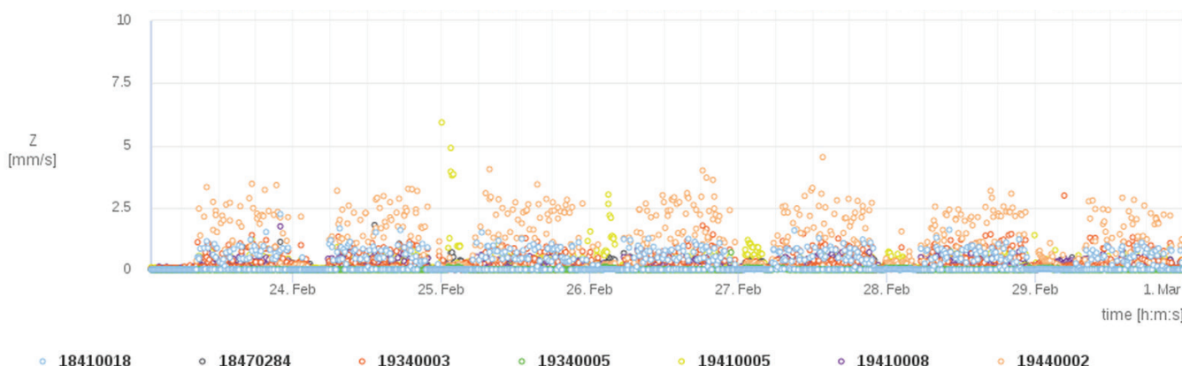
Figure 9. Relevé hebdomadaire des 7 balises de l'axe de mesure vertical, aucune amplitude supérieure à 7mm/s, semaine conforme à l'IN1226.
